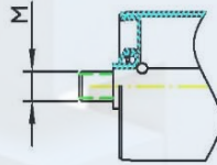
REM (ROSCA EXTERIOR MÉTRICA)
