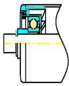
LIS (EJE LISO)
