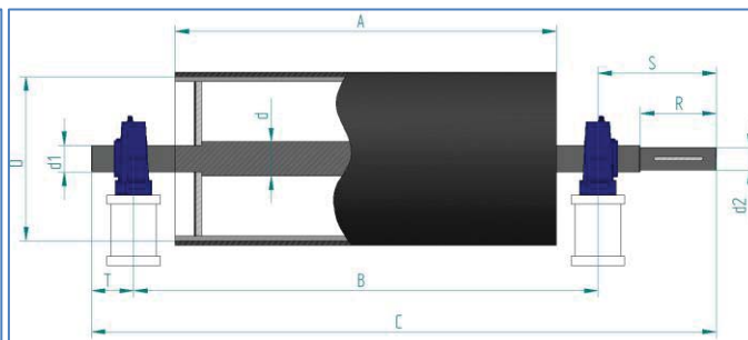
Eixo soldado
